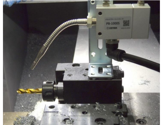
パルスブロー(PB-1000S) + フレキシブルノズル(PB-FN150)
